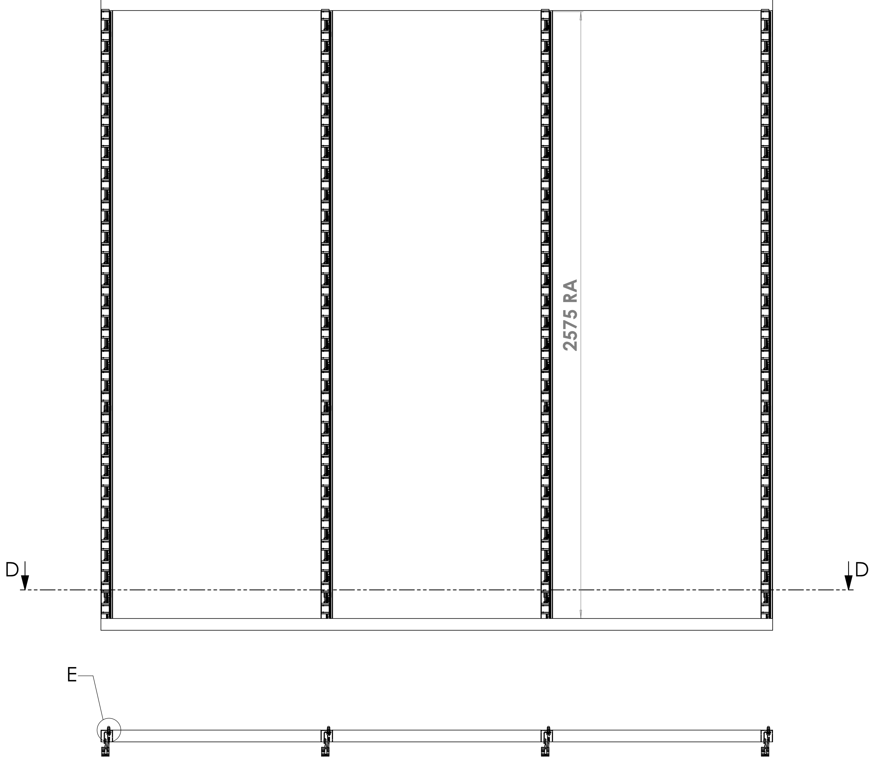
SECTION D-D
